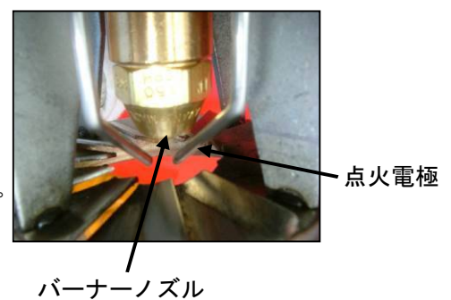
【バーナーノズル部詳細】
