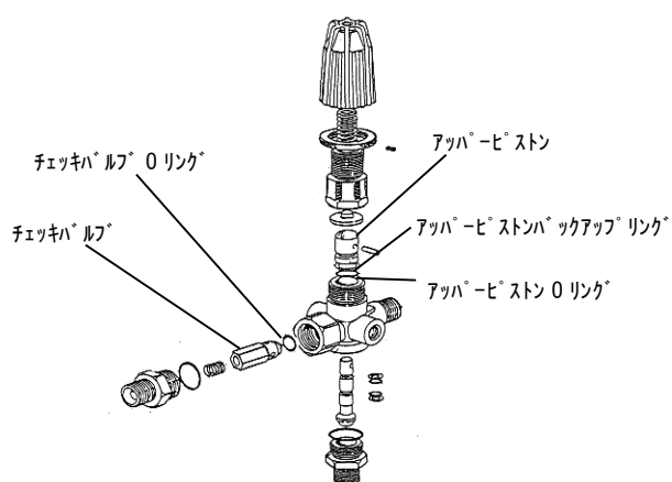
圧力調整弁(アンロードバルブ)
