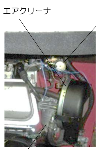
エアクリーナ 気化器 (キャブレター)
